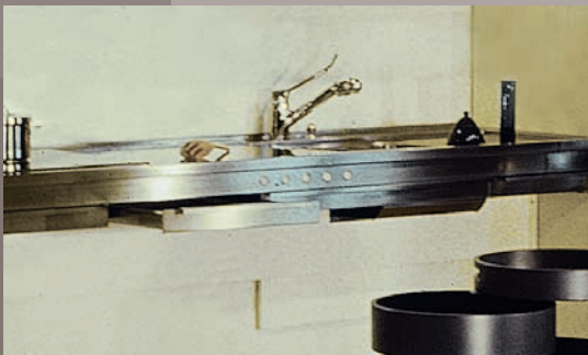
Küche im Privathaushalt mit höhenverstellbarem Koch- / Spültisch und absenkbarem Oberschrank
